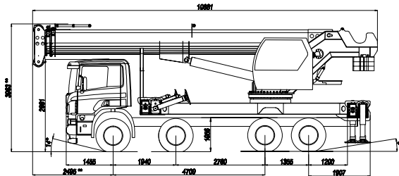
TRUCK: SCANIA P380 CB 8X4 EHZ CRANE : HK 90 22 T2
